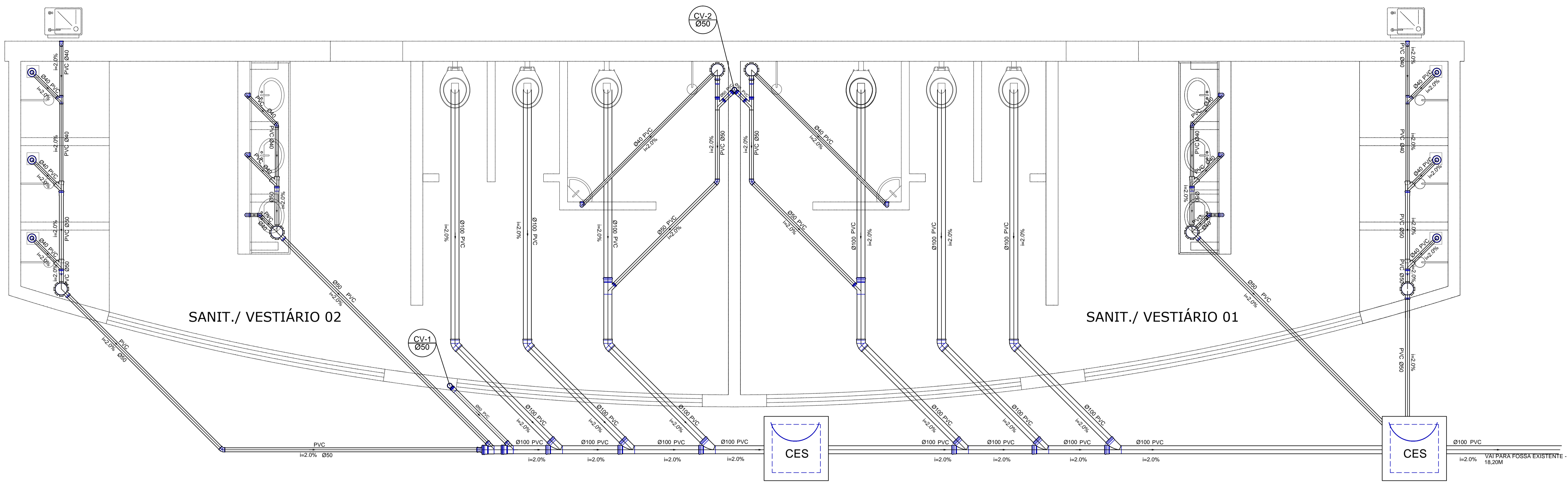
Planta - Esgoto Sanitário escala 1:25
