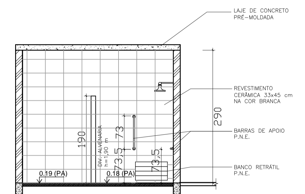
VESTIÁRIO: VISTA D ESCALA 1:50
