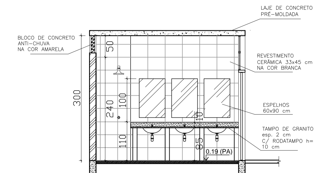
VESTIÁRIO: VISTA A ESCALA 1:50
