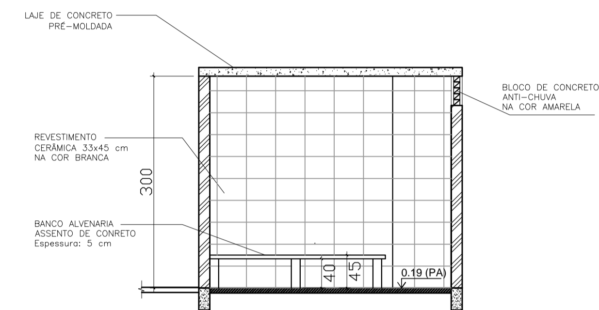
VESTIÁRIO: VISTA B ESCALA 1:50
