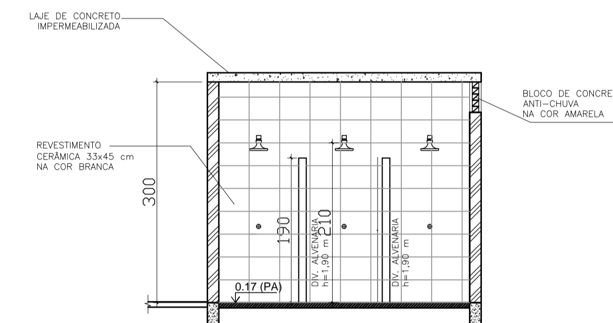
VESTIÁRIO: VISTA C ESCALA 1:50
